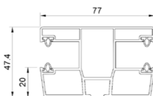
Guía dividida (PVC) - Revisión RS desde el interior. MK939
