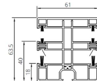
Guía (PVC) de doble cara + MKT*. R0004
