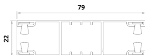
Guía doble cara (para lamelas H37 y H42). 87858
