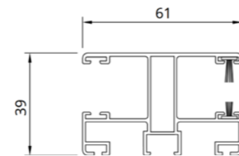
Guía (ALU) de una / de doble cara
