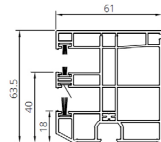
Guía (PVC) de una cara + MKT*. R0003
