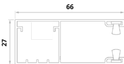
Guía de una cara (para lamelas H55). PP6600
